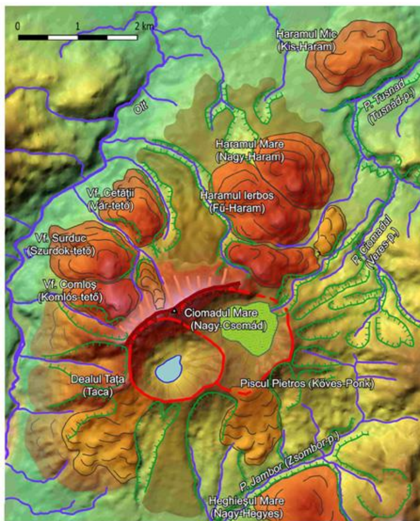
A dél-hargitai Csomád vulkánmorfológiai térkép vázlatja
